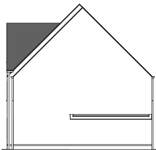
Zijgevel rechts
