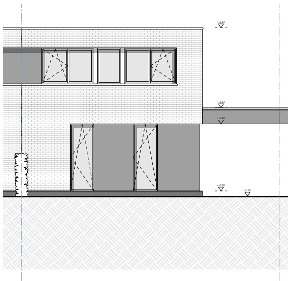
Vorgevel
