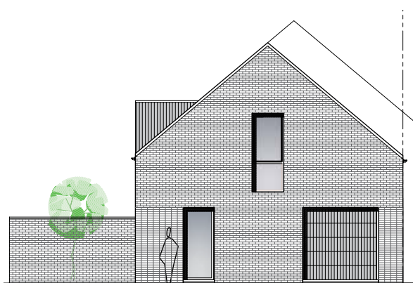
Vorgevel
