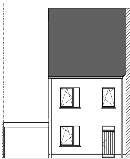
Vorgevel
