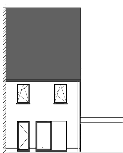
Achtergevel
