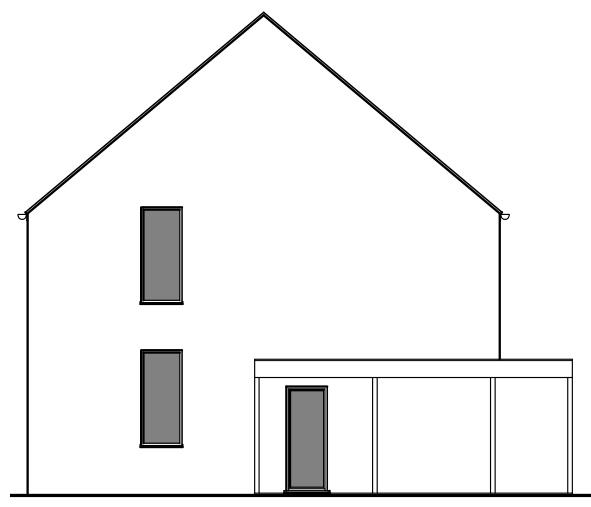
Zijgevel rechts
