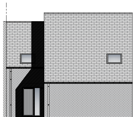
Zijgevel rechts
