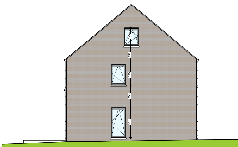
Façade latérale gauche
