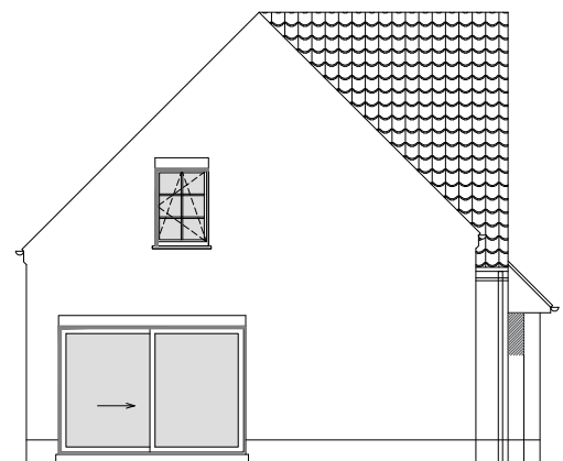
Zijgevel links
