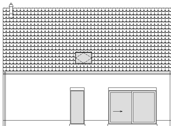
Achtergevel
