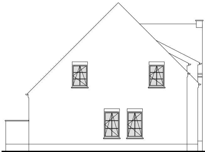
Zijgevel links
