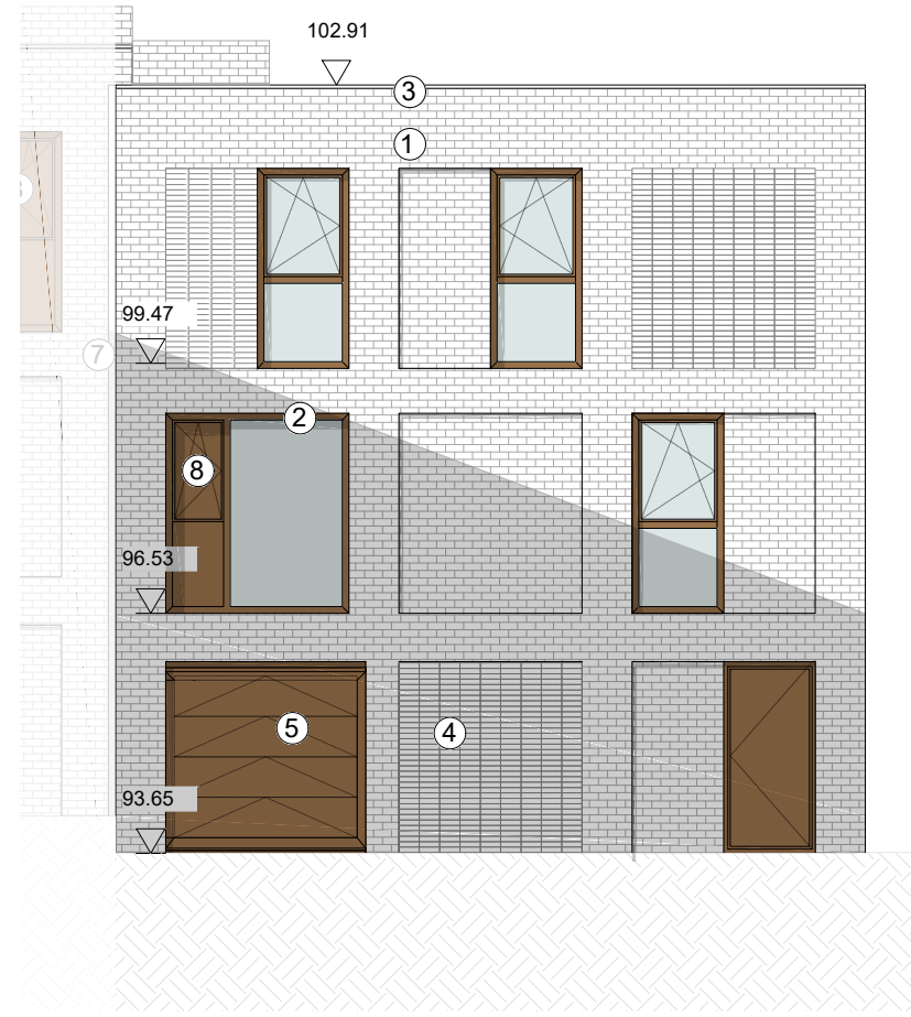
Façade nord-est / côté rue Noordoost gevel / straat kant
