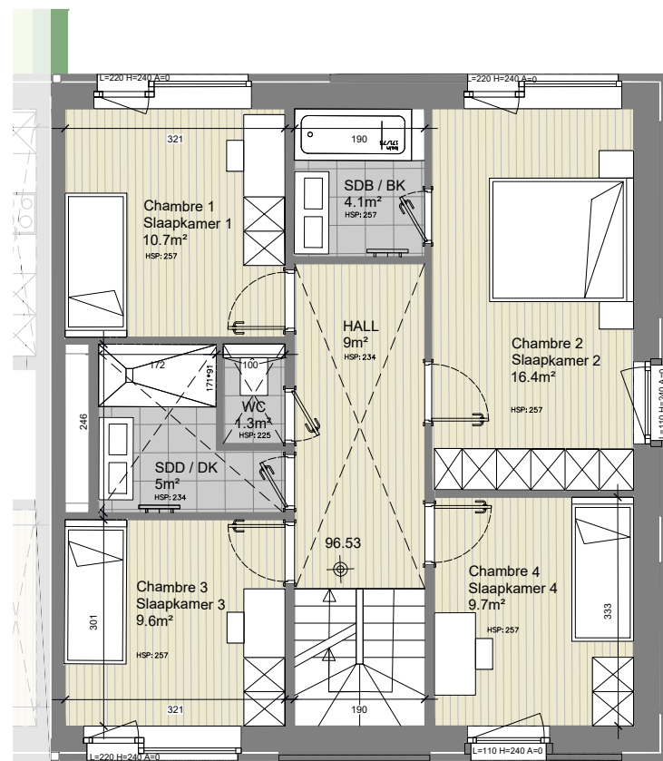
Premier étage / Eerste verdieping
