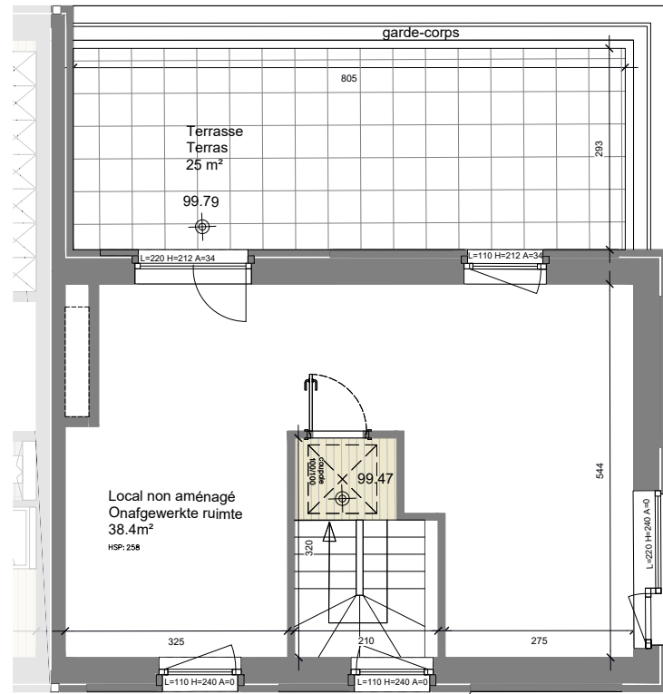
Deuxième étage / Tweede verdieping
