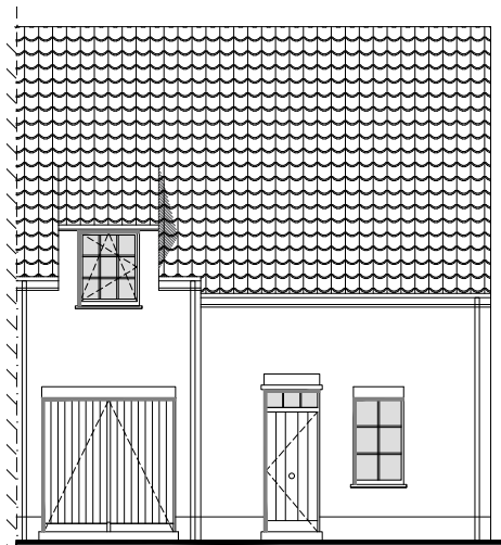
Voorgevel
