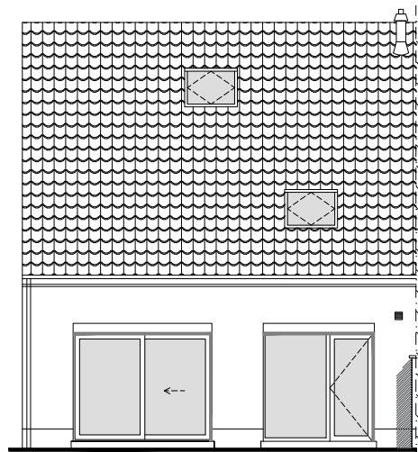
Achtergevel
